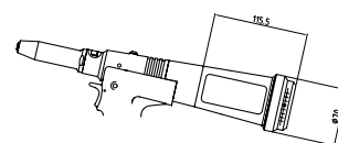
Opción de vaso recoge-clavos fijo (serie 71204)
